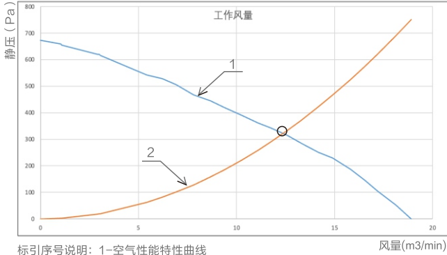
标序号说明：1—空气性能特性曲线 2—排烟阻力曲线 ○—工作点
